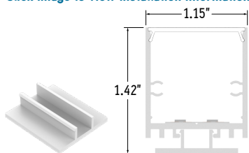
Mounting Clip (LLED8650-WRC-MC)
